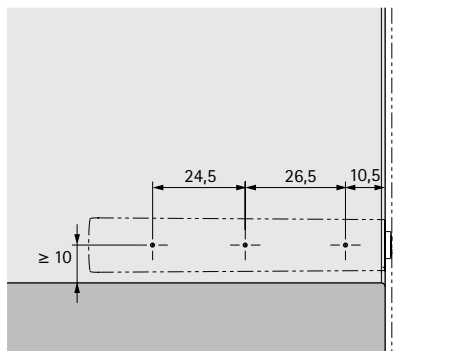
Карта сверления для длинного хода, накладная и вкладная навеска
